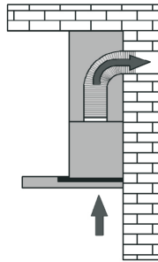
(мал. 1. Відвід)
