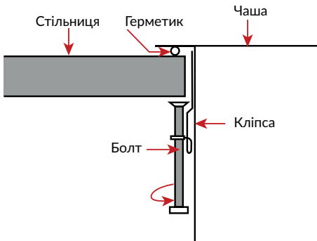
Врізний монтаж
