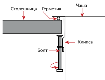
Врезной монтаж
